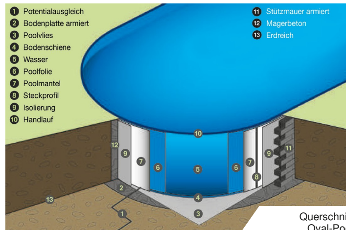
vollversenkt
