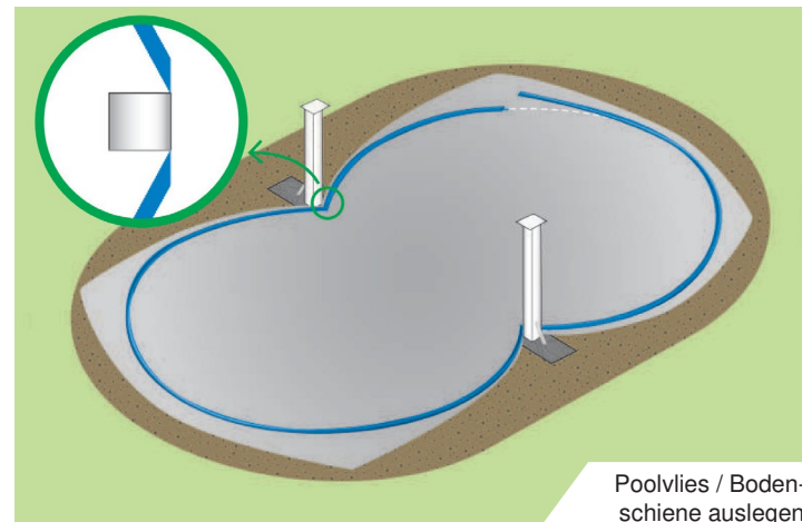
Aufbau Stützkonstruktion
