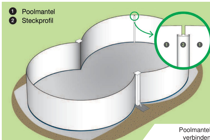
Poolmantel aufstellen
