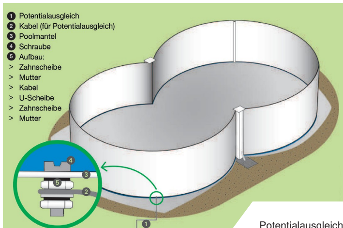
Potentialausgleich
